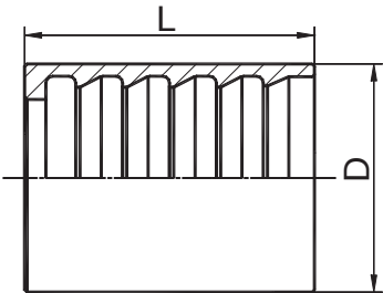
KF00110 SAE100R1AT/EN 853 1SN 软管套筒 FERRULE FOR SAE100R1AT/EN 853 1SN HOSE
